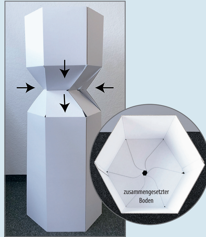
2. Falz nach Innen drücken bis sich die einzelnen Abschnitte miteinander verhaken, dann nach unten drücken
