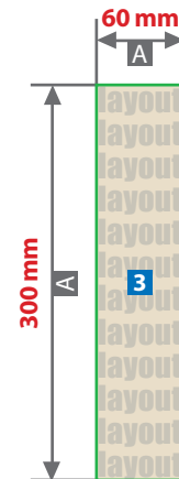
Druckbereich 3 Ärmel (links/rechts)
